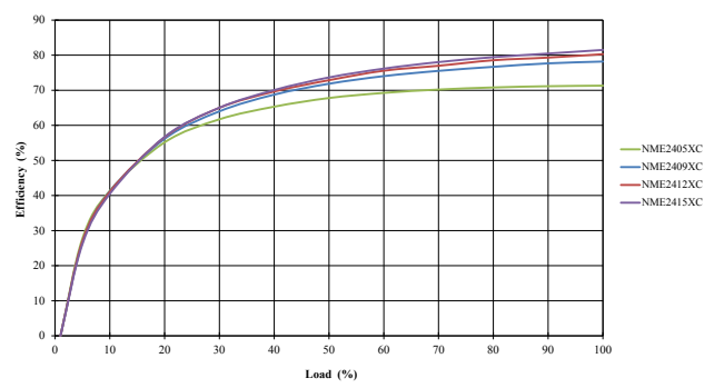
24V Inputs
