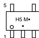
TSOP-5
