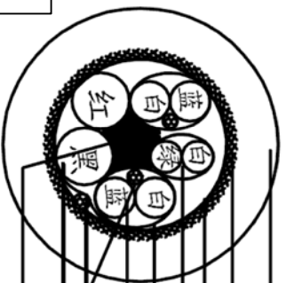
DETAIL A-A
