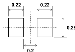
Fig. 10.3.1 (Unit: mm)
