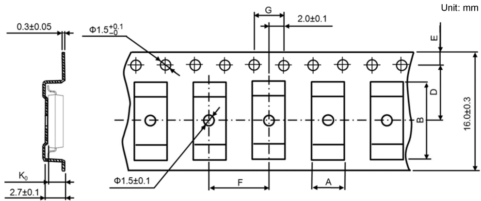
Fig. 16.3.4.1 Tape dimension
