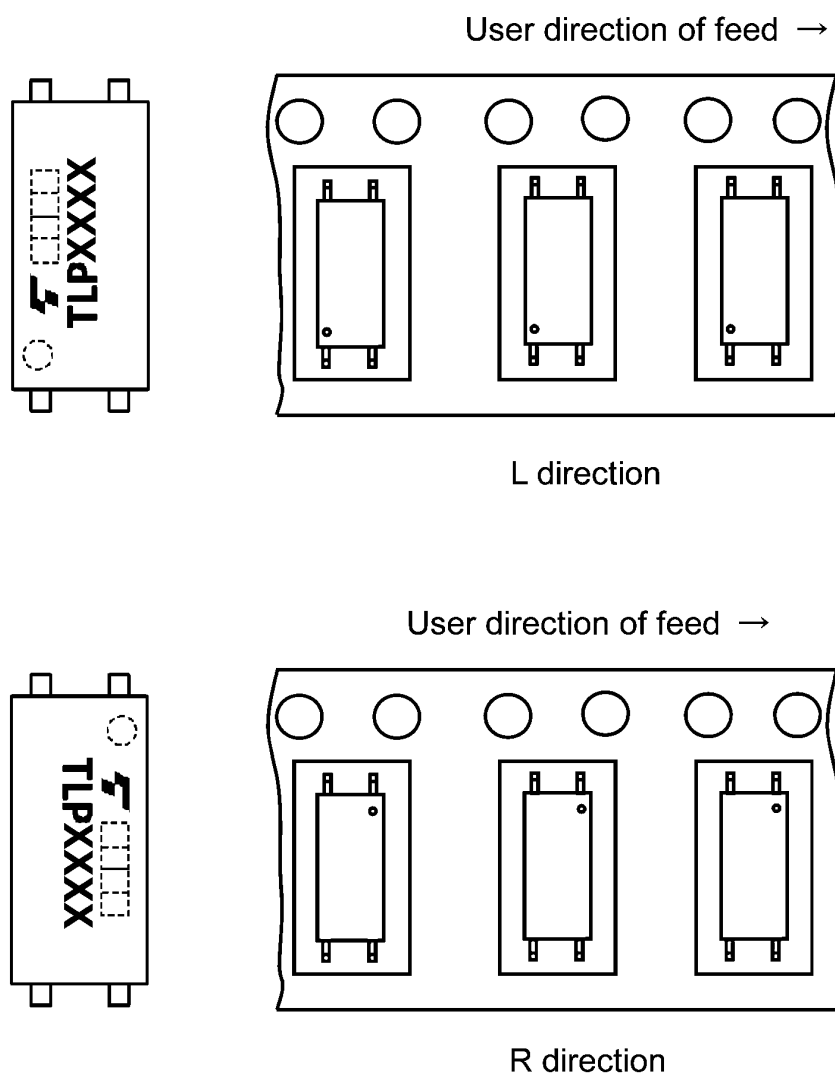
Fig. 16.3.1.1 Device Orientation
