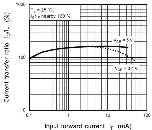
Fig. 11.12 I_C/I_F - I_F
