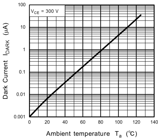
Fig. 11.9 I_{DARK} - T_a
