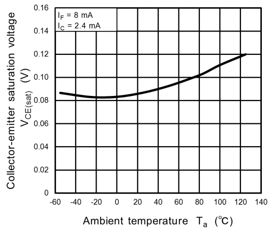
Fig. 11.10 V_{CE(sat)} - T_a
