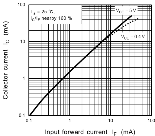
Fig. 11.11 I_C - I_F
