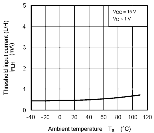
Fig. 13.2.4 I_{FLH} - T_a
