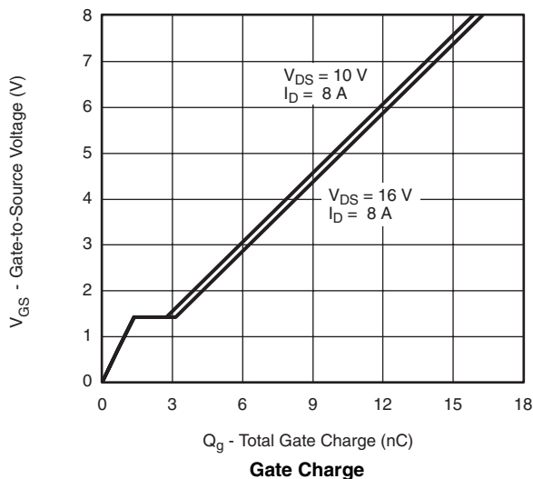
V_{DS} = 10\text{ V} I_D = 8\text{ A} V_{DS} = 16\text{ V} I_D = 8\text{ A} Gate Charge
