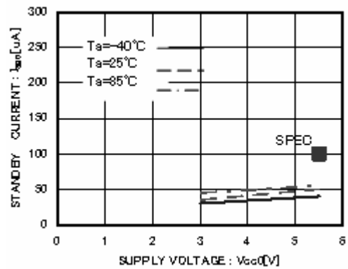
Figure 21. Standby Current0 I_{St0}
