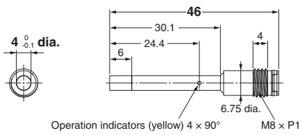
E2E-S05N03-MC-□□
